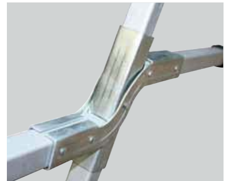
Zusätzliche Verstärkungen im Beinbereich.
