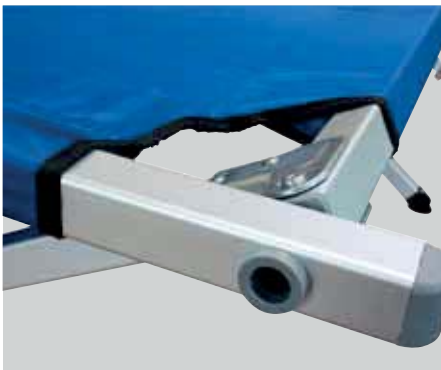
Dreifach vernähter, doppelagiger Bezug an allen Reibungspunkten.
